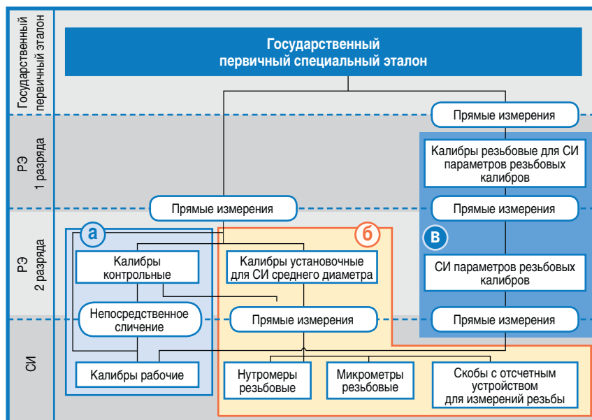
Рис. 3 Общая структура поверочной схемы для средств измерений параметров резьбы
