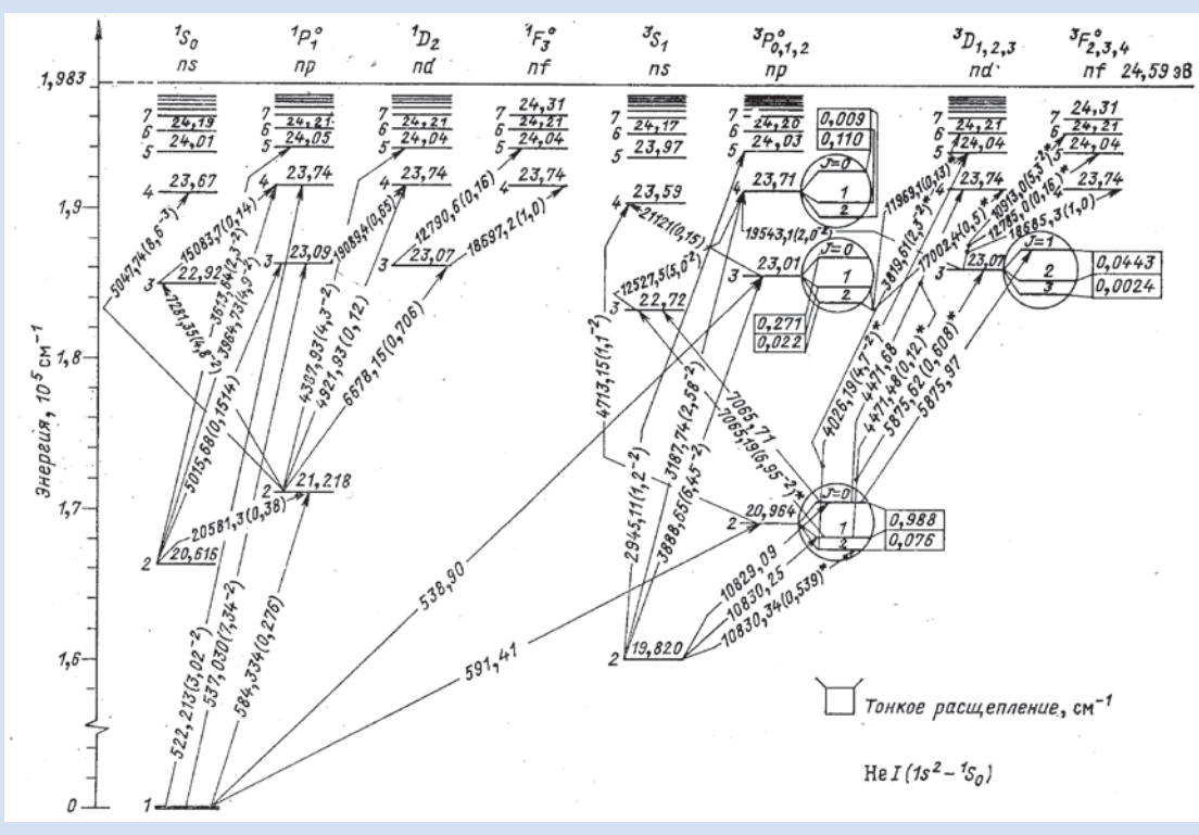
Рис. 2 Диаграмма Гроттриана для атома гелия
