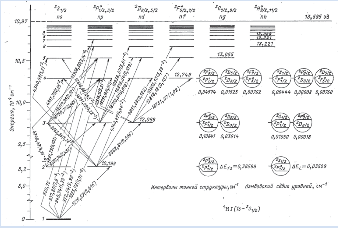
Рис. 1 Диаграмма Гроттриана для атома водорода
